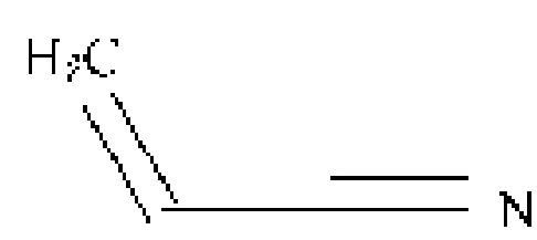
图 A.1 丙烯腈标准品的结构式
