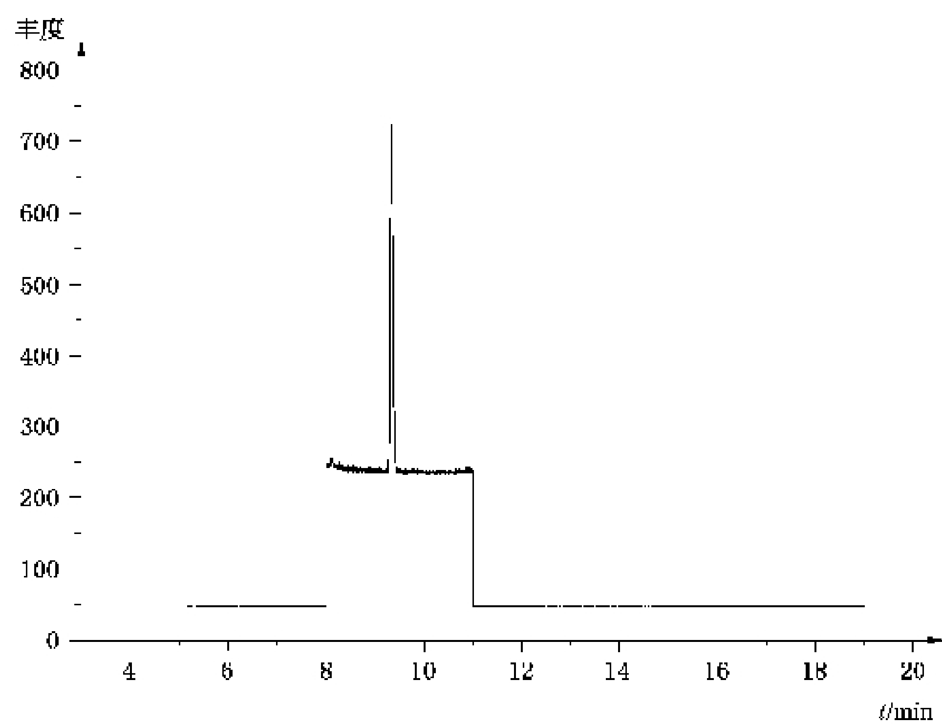
图 A.2 丙烯腈标准品选择离子色谱图
