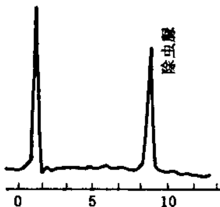
图 1 除虫脲的标准色谱图
