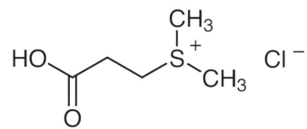
图 1 (2-羧乙基) 二甲基氯化硫的结构式
