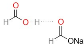
图1 二甲酸钠的结构式
