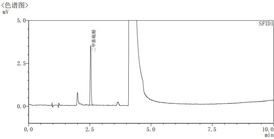
图 D.1 二甲基硫醚标准工作溶液（4 μg/mL）气相色谱图
