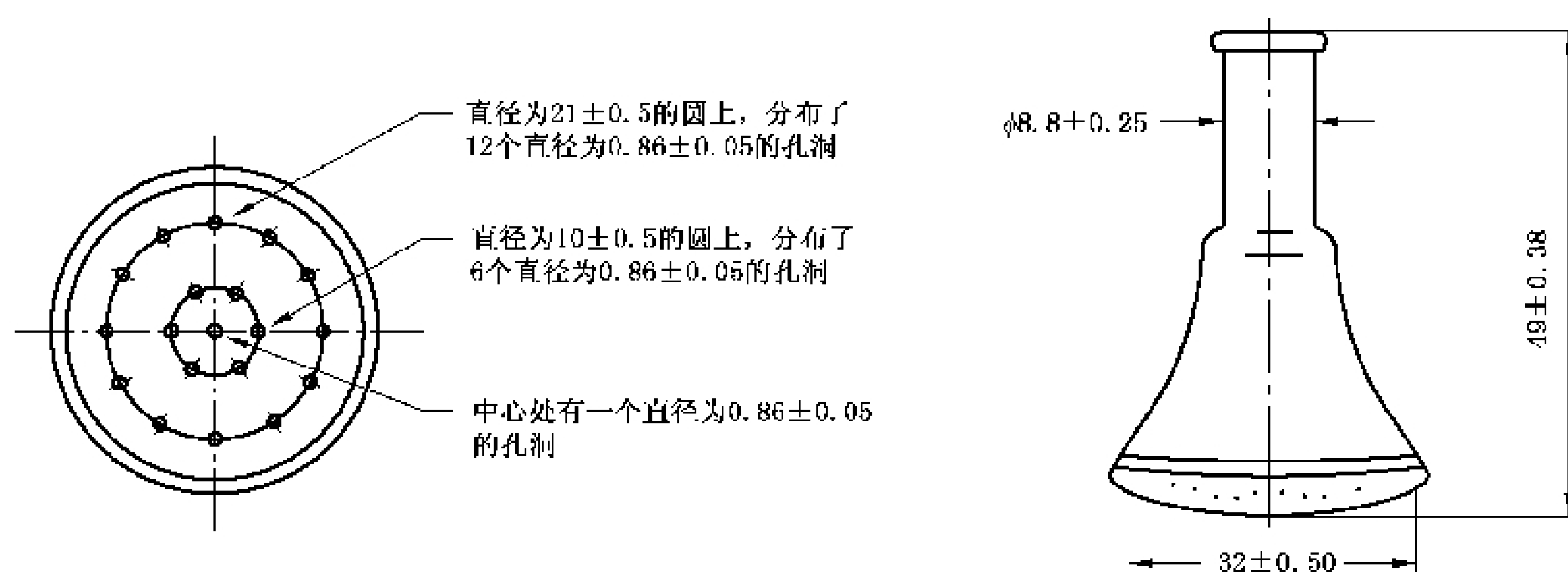
图2 喷淋实验装置中的喷淋喷嘴
