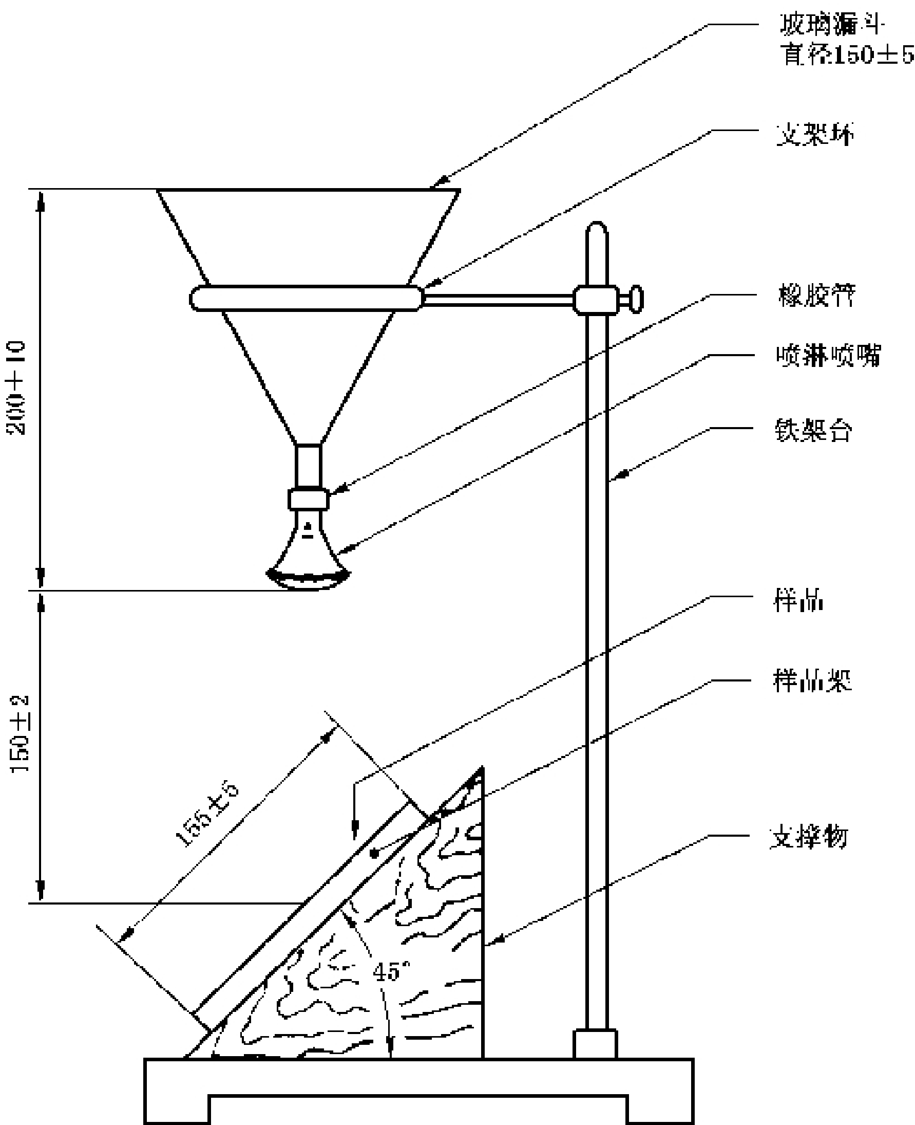
图 1 喷淋实验装置详细图
