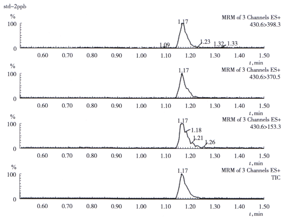
图 B.1 氯酯磺草胺标准溶液 LC-MS/MS 的多反应监测(MRM)图
