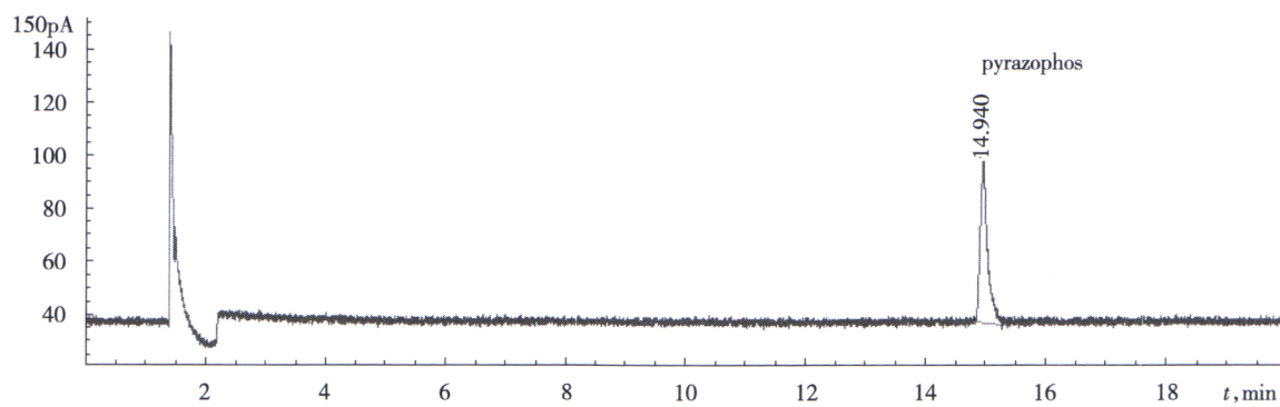
图 A.1 吡菌磷标准品气相色谱图
