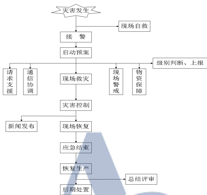
图A.1 雷电灾害应急响应程序框图
