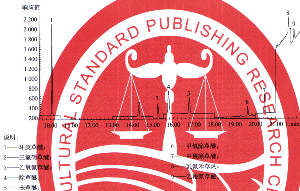
图 B.1 二苯醚类除草剂标准溶液总离子流色谱图
