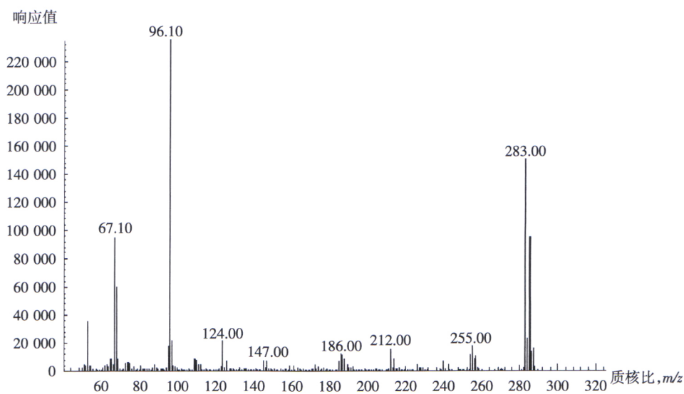
图 A.4 腐霉利标准品的质谱图
