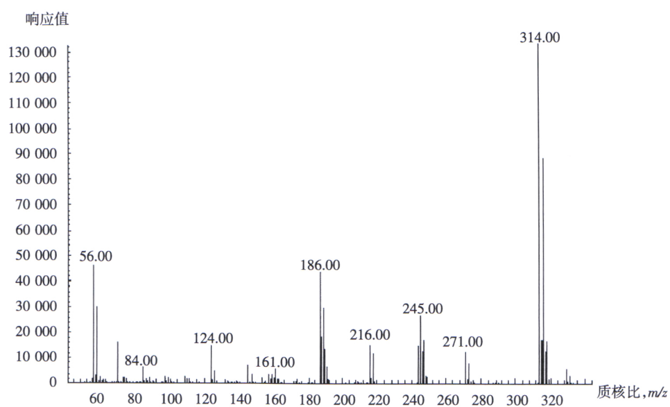
图 A.5 异菌脉标准品的质谱图
