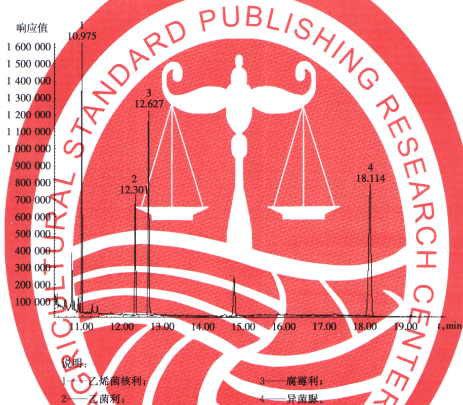
图 A.1 乙烯菌核利、乙菌利、腐霉利、异菌脲标准品总离子流色谱图
