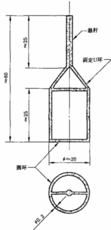
图 1 圆环尺寸示意图
