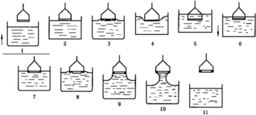
图 B.2 测量表面张力示意图
