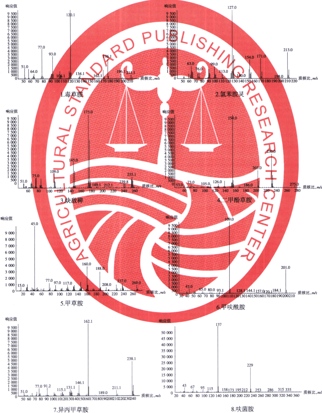
图 C.1 25 种苯酰胺类农药标准品质谱图
