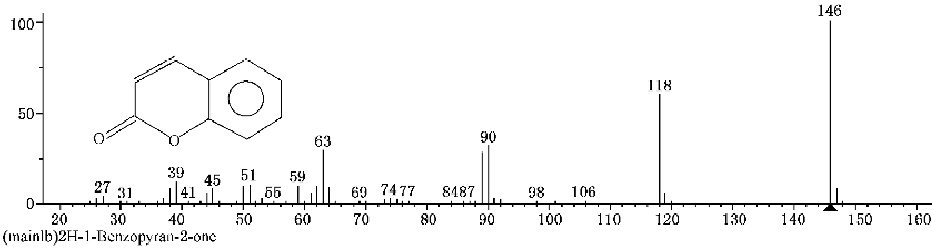
图 C.5 香豆素标准物质的质谱图
