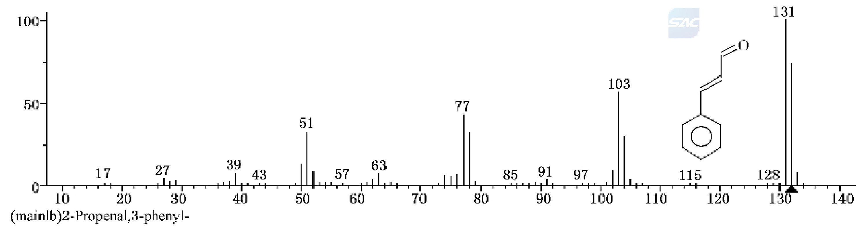
图 C.4 肉桂醛标准物质的质谱图
