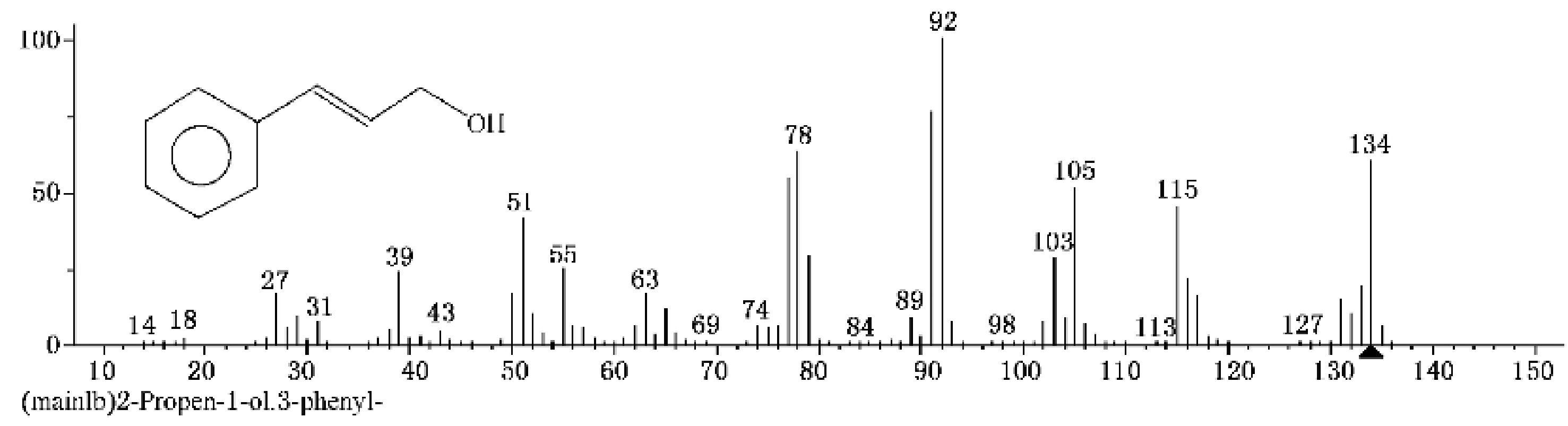
图 C.2 肉桂醇标准物质的质谱图
