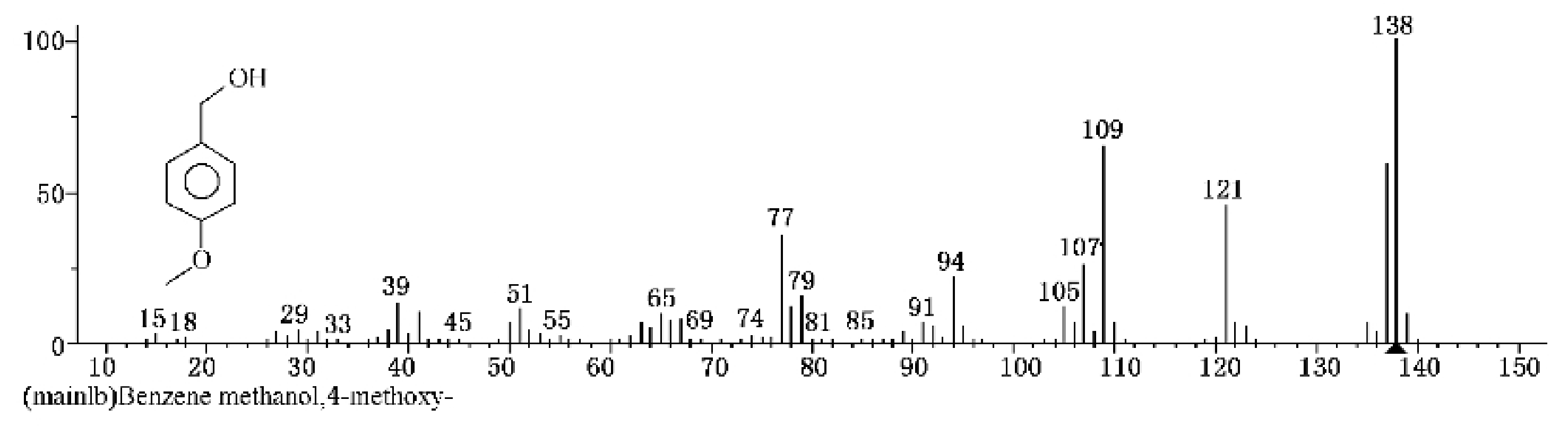
图 C.3 茴香醇标准物质的质谱图
