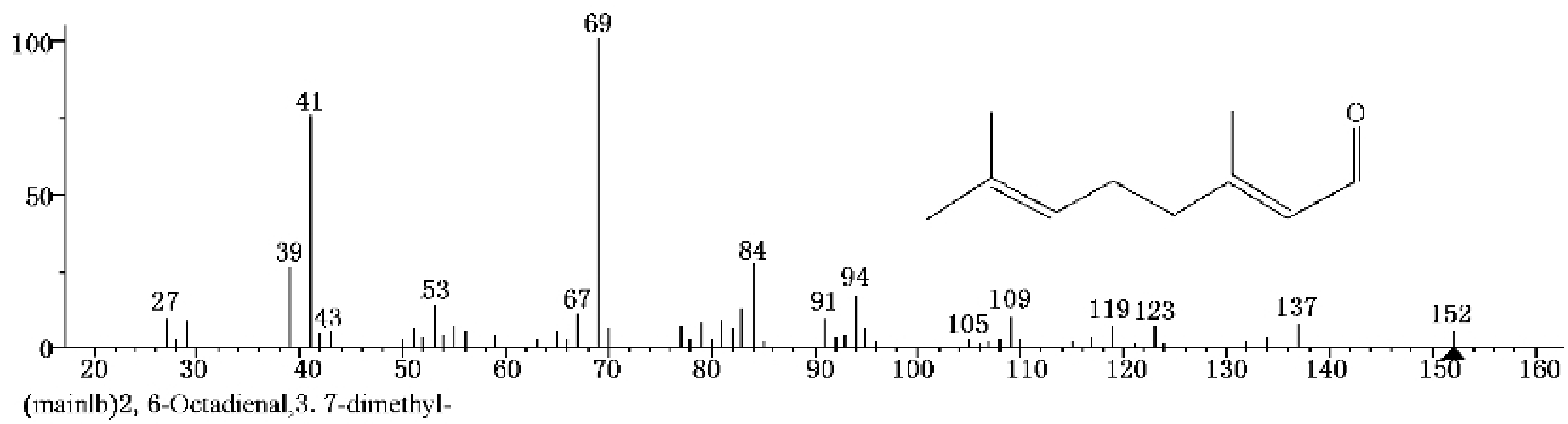
图 C.1 柠檬醛标准物质的质谱图
