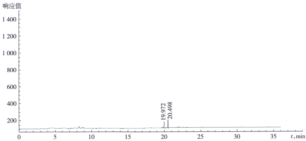
图 B.4 花生空白样品气相色谱图
