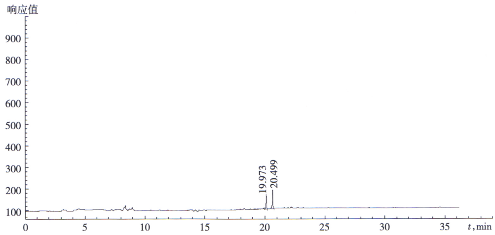
图 B.3 小豆空白样品气相色谱图
