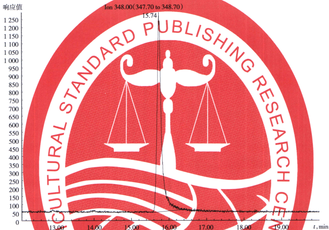
图 A.1 苯醚甲环唑标准溶液( 0.1\ \mu\text{g}/\text{mL} )GC-MSD/NCI 选择离子流色谱图
