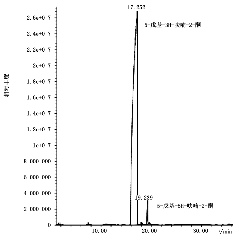
图 B.1 食品添加剂 5-戊基-3H-呋喃-2-酮气相色谱图
