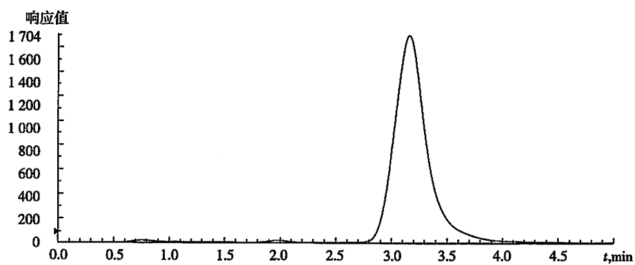
图 1 0.01 \mu\text{g/mL} 灭瘟素标准溶液色谱图
